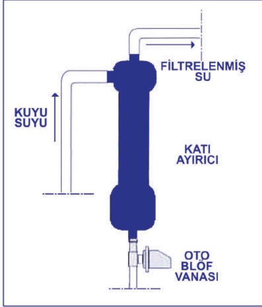
AquaTROL Katı Ayırıcı Uygulama Örneği
